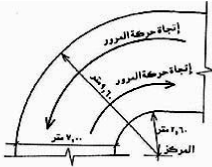
شكل رقم (٥) مسقط أفقي يوضح منحنى ذا اتجاهين لحركة المرور
